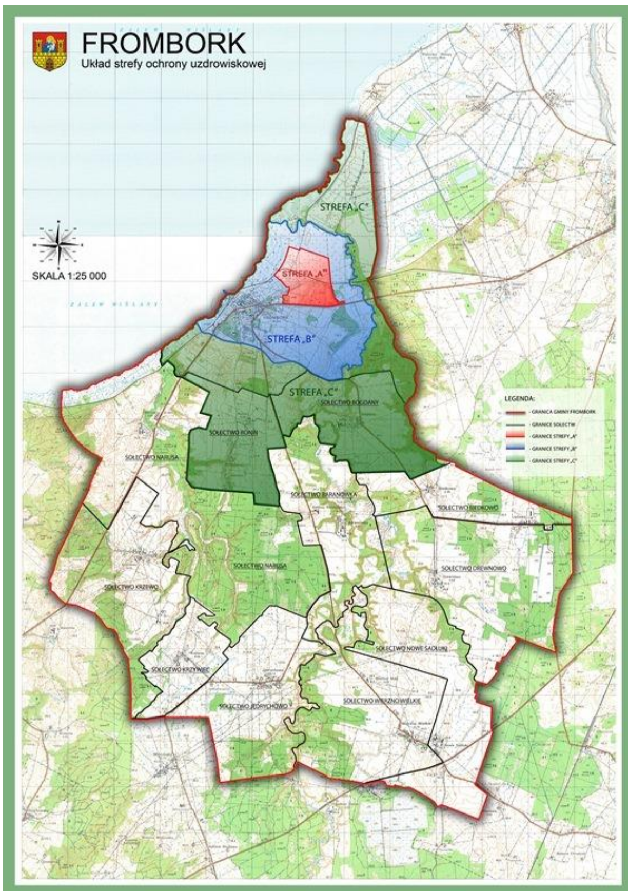
Strefy A, B i C ochrony uzdrowskiej wg. Decyzji Ministra Zdrowia Nr 68 z dnia 25.03.2013r.
